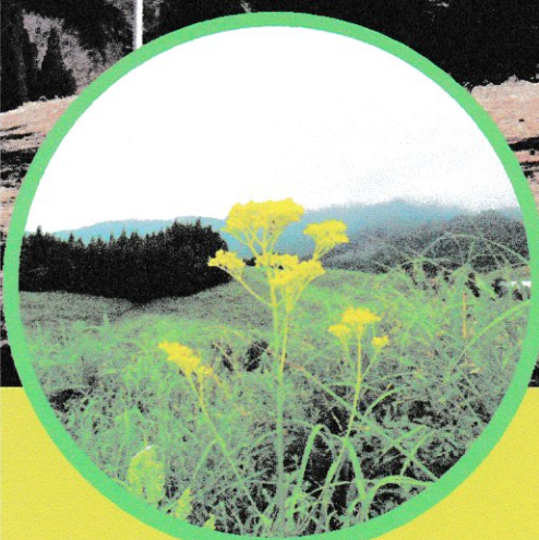
オミナエシ
